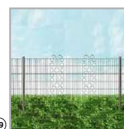
Typ R-S O-2 mit zwei Zierelementreihen Maschenweite 50 x 200 mm
