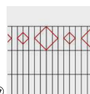
Dekor Karo Typ II je Schmuckzaunelement 6 Stück Karos Ø 185 mm 5 Stück Karos Ø 90 mm
